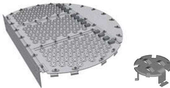
Рис. 1. Клапанні тарілки EDV
