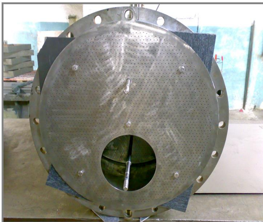
Рис. 2. Тарілка із змінним живим перерізом
