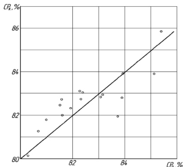
Рис.1. Зміна масової ділі сухих речовин між кристалльного розчину при нагріванні потоку утфелю в електричному нагрівачі
