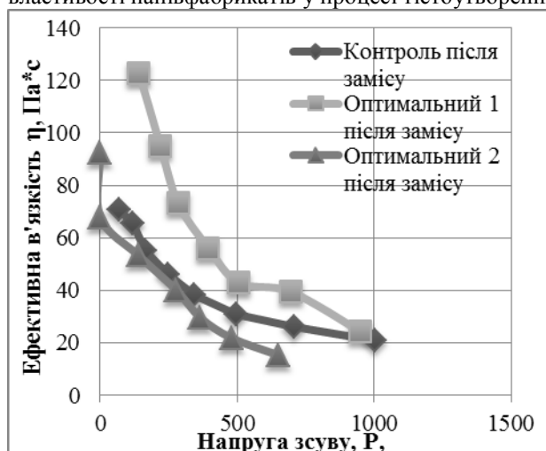
Рис 4. Крива в'язкості тіста після замісу
