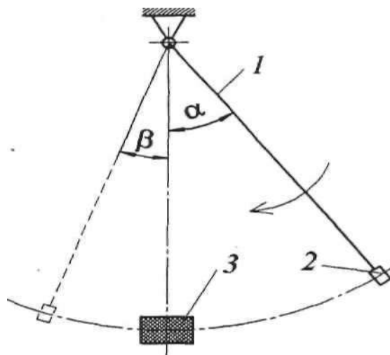
Рис. 1. Схема установки для дослідження процесу різання:
