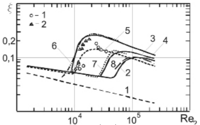
Рис.3. Залежність \xi = f(Re_2) при \Gamma_v = 0,5 \cdot 10^{-3} м 2 /с.
