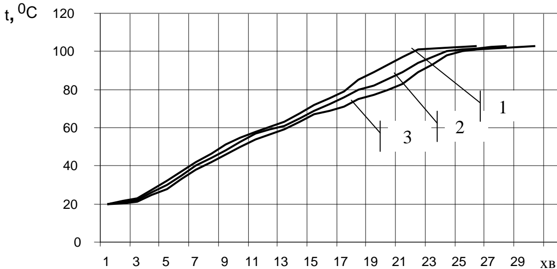
Рис 1. Кінетика випікання кексів на різних видах борошна: 1– пшеничному та рисовому, 2– кукурудзяному, 3–гречаному
